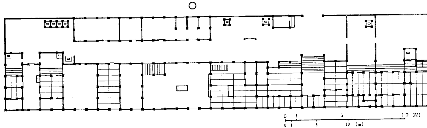
図7-1 タイプAの例：「江戸本郷邸年寄中之小屋（加越能文庫）」より 原図には、小者部屋・徒者部屋・拾人部屋等の部屋名、天井や窓の仕様、ナガシ・セッチン・イロリ等の書込がある。 大鋸コレクションほど詳細に描かれておらず、柱割や畳の敷き方等、起こす時に補った箇所も多い。
