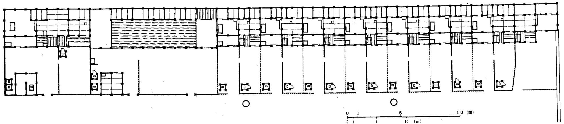
図7-3 タイプDの例：「東御長屋上壇（大鋸コレクション）」より 図7-2同様、原図は非常に詳細な絵図である。左から二番目の、間口10間程の部分は「武芸稽古所」と書かれており、江戸御上屋敷 絵図とは異なっている。数箇所明らかに合理性を欠くところがあり、それについては図を起こす際に類推して変更してある。
