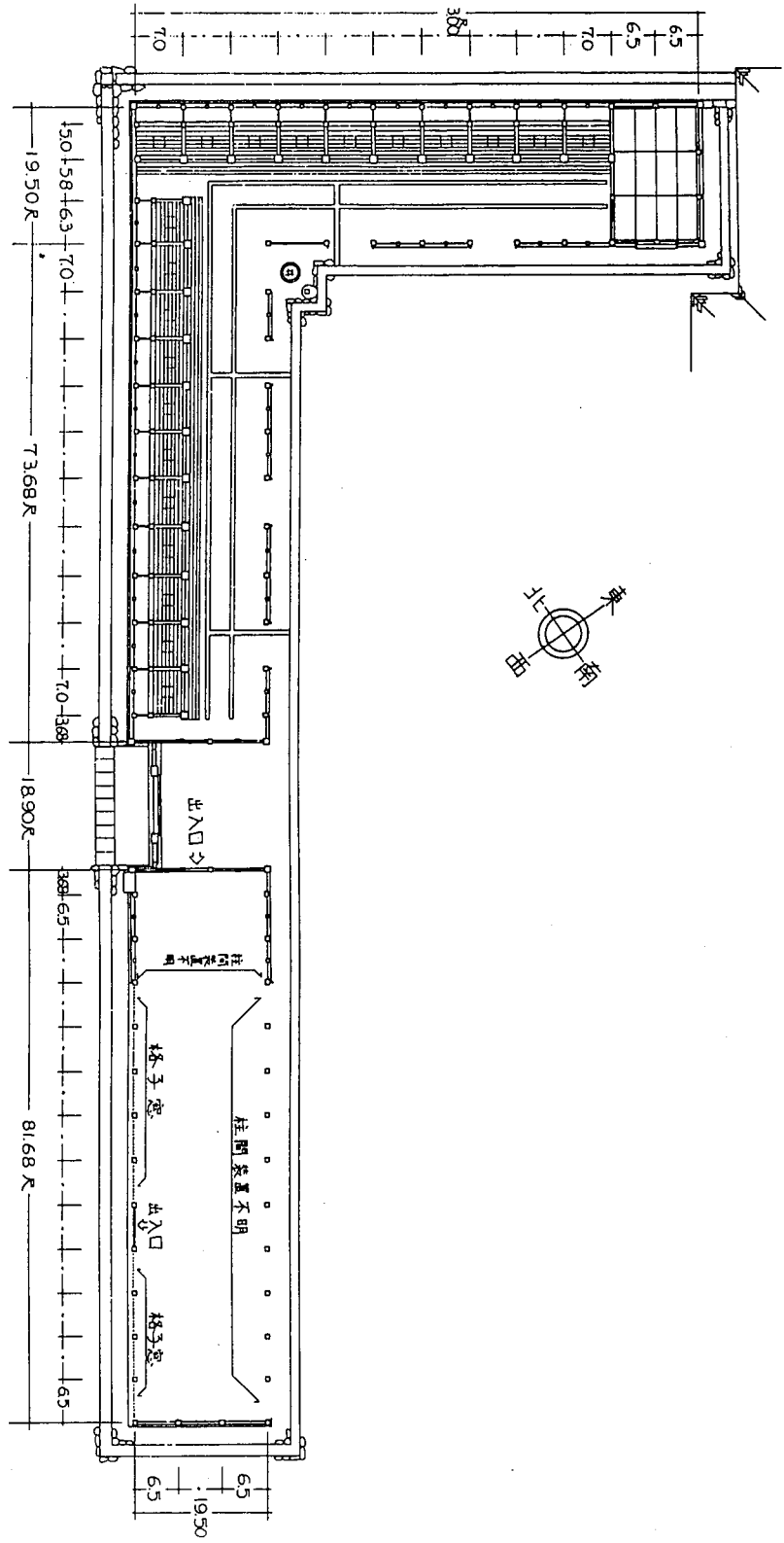
図 6 当初全体平面図 (『重要文化財形根城馬屋等修理工事報告書』より)
