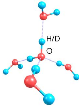
図1 水分子とその水素結合
