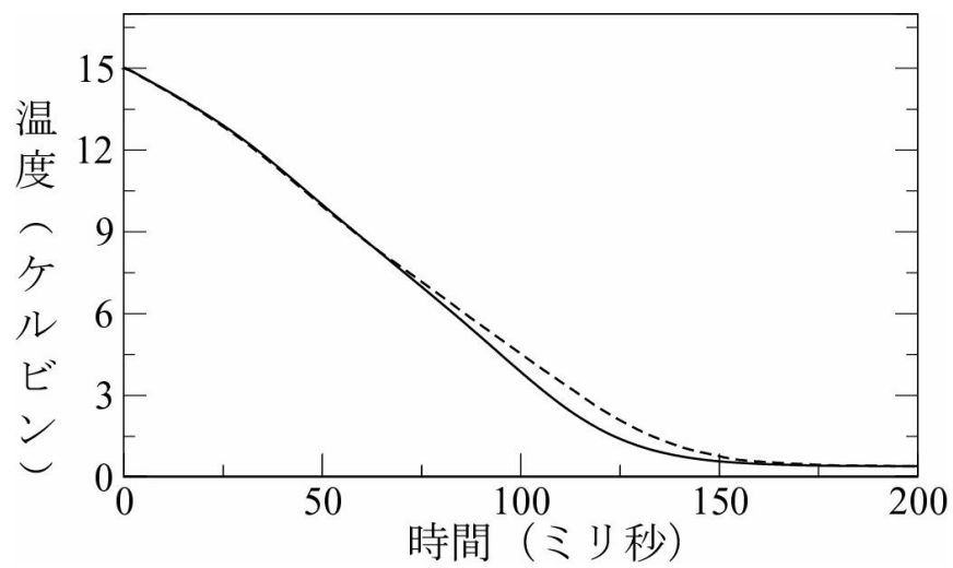
図2 励起状態に生成された反水素原子の温度の蓄積時間依存性
