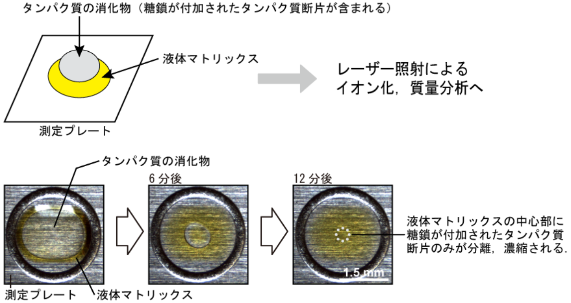
図 1. 液体マトリックスを用いた新規の MALDI 質量分析法
