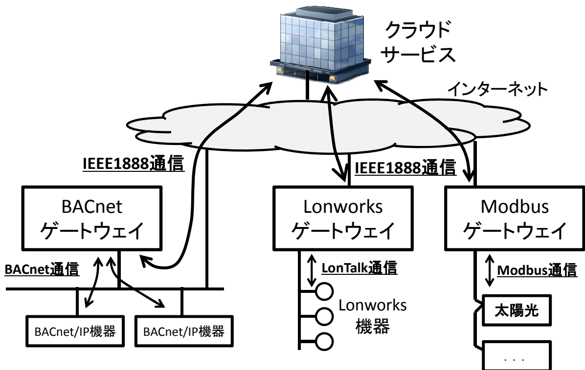
図 1：BACnet/Lonworks/Modbus ゲートウェイ機器の模式図
