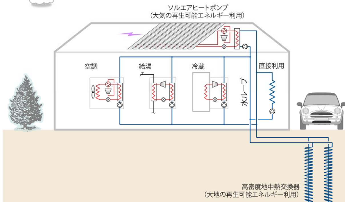
図1 システム構成例（住宅への適用イメージ）
