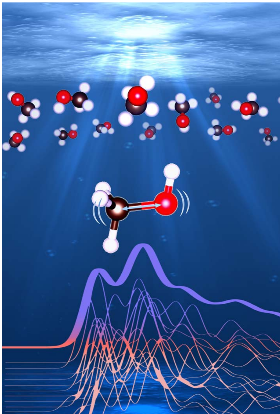
図1 本研究成果の模式図。液体メタノールのスペクトルからメタノール分子の動的挙動の情報を調べることができる。
