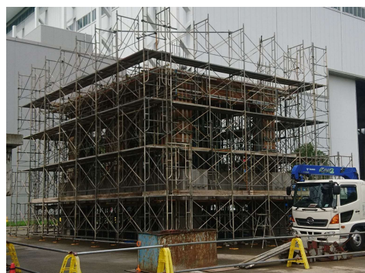
写真 試験体の施工状況
