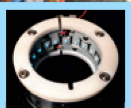
紫外線発光ダイオード(UV-LED)を用いたリングモジュール水消毒装置(特許第6208563号)
