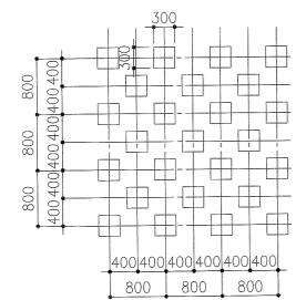
①部詳細図 1:60
