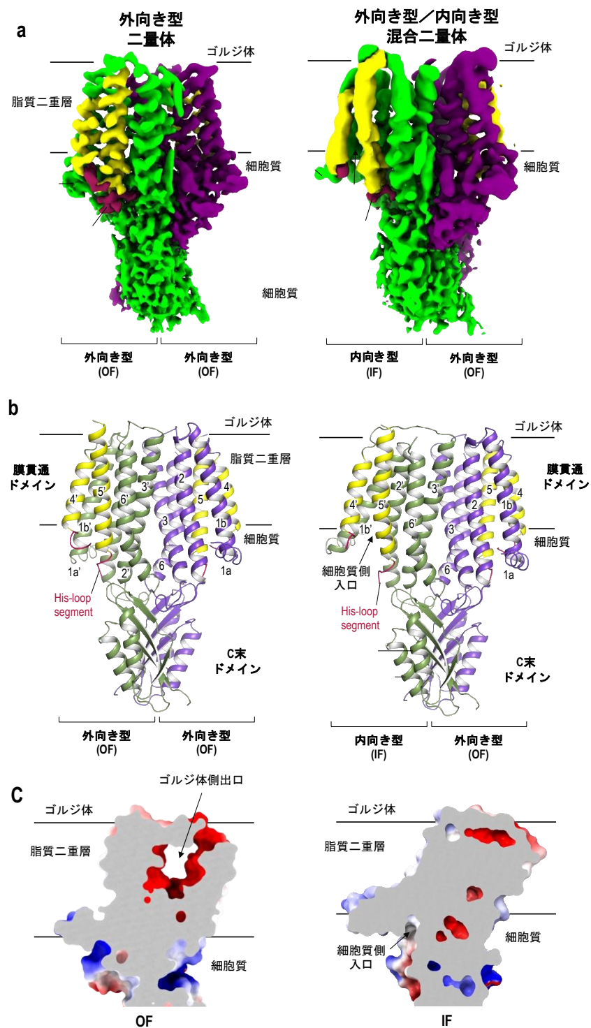
図 1. ZnT7 二量体のクライオ電子顕微鏡マップ (a)、分子構造モデル (b)、静電電荷マップの断面図 (c)。 外向き型構造では、ゴルジ体側に垂鉛を放出する出口が形成される。一方、内向き型構造では、細胞質側から垂鉛を取り込むための入口が形成される。
