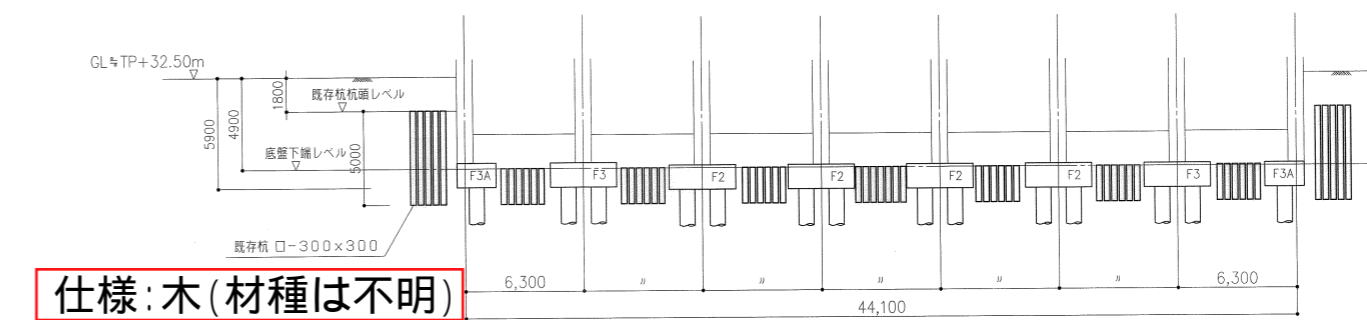
ア-ア 断面図 1:200
