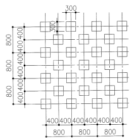
①部詳細図 1:60
