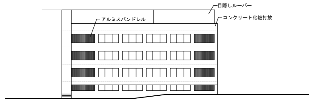
東側立面図
