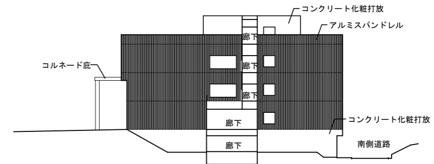
北側立面図
